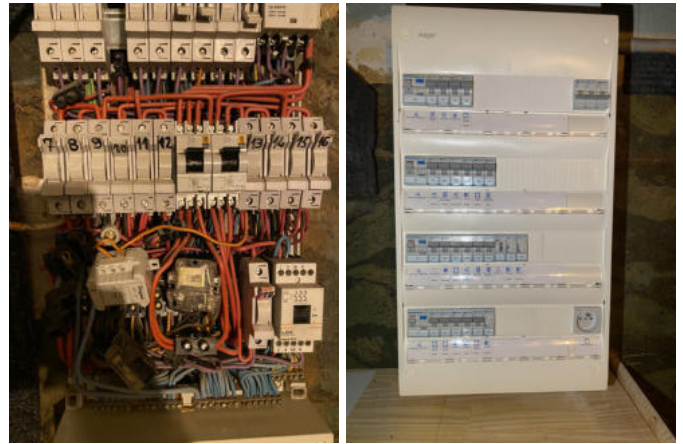
Rénovation d'un tableau électrique Avant/Après
